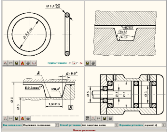
Элементы установки колец
