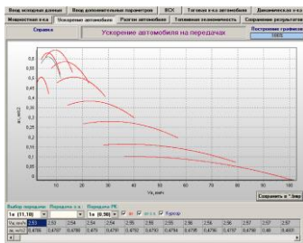
Окно расчета ускорения
