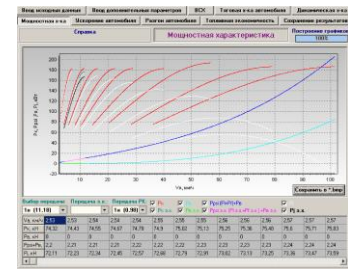
Окно расчета характеристик двигателя
