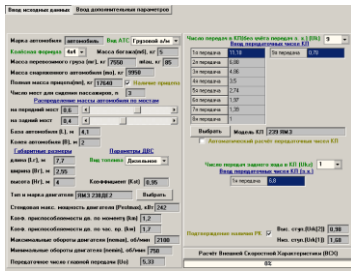
Головное окно программы Расчета тяговой динамики
