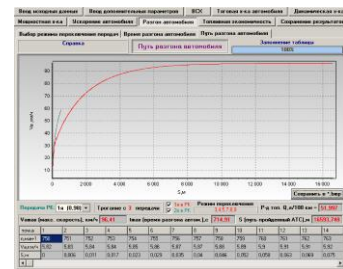
Окно расчета зависимости скорости от пути
