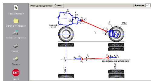
Схема карданных валов
